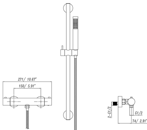
Schemat wymiarów [mm / cale]:
