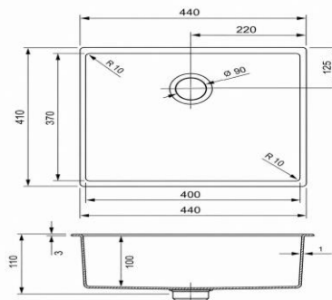
Zlewozmywak dla osób niepełnosprawnych LEX02-11
